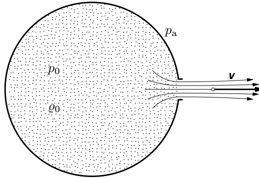
Obr. 22 Adiabatický výtok plynu z tlakové nádoby
