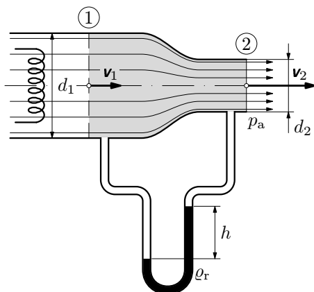
Obr. 24 Difuzor opalovače
