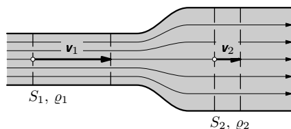
Obr. 19 K rovnici kontinuity pro plyny
