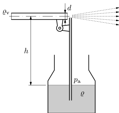
Obr. 22 Rozprašovač
