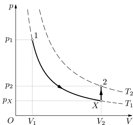
Obr. 3 K odvození stavové rovnice
