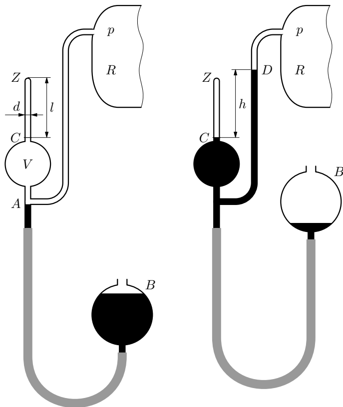
Obr. 12 McLeodův vakuometr
