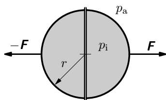
Obr. 10 Magdeburské polokoule
