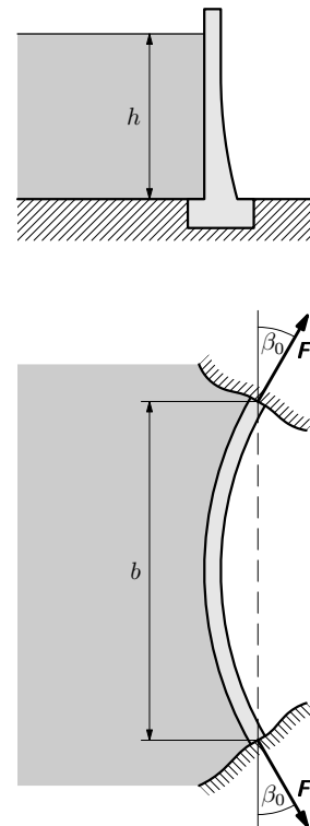
Obr. 43 Klenbová hráz údolní přehrady
