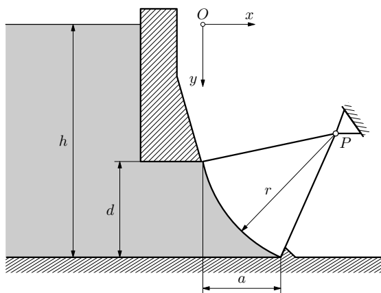
Obr. 41 Schéma segmentového stavidla
